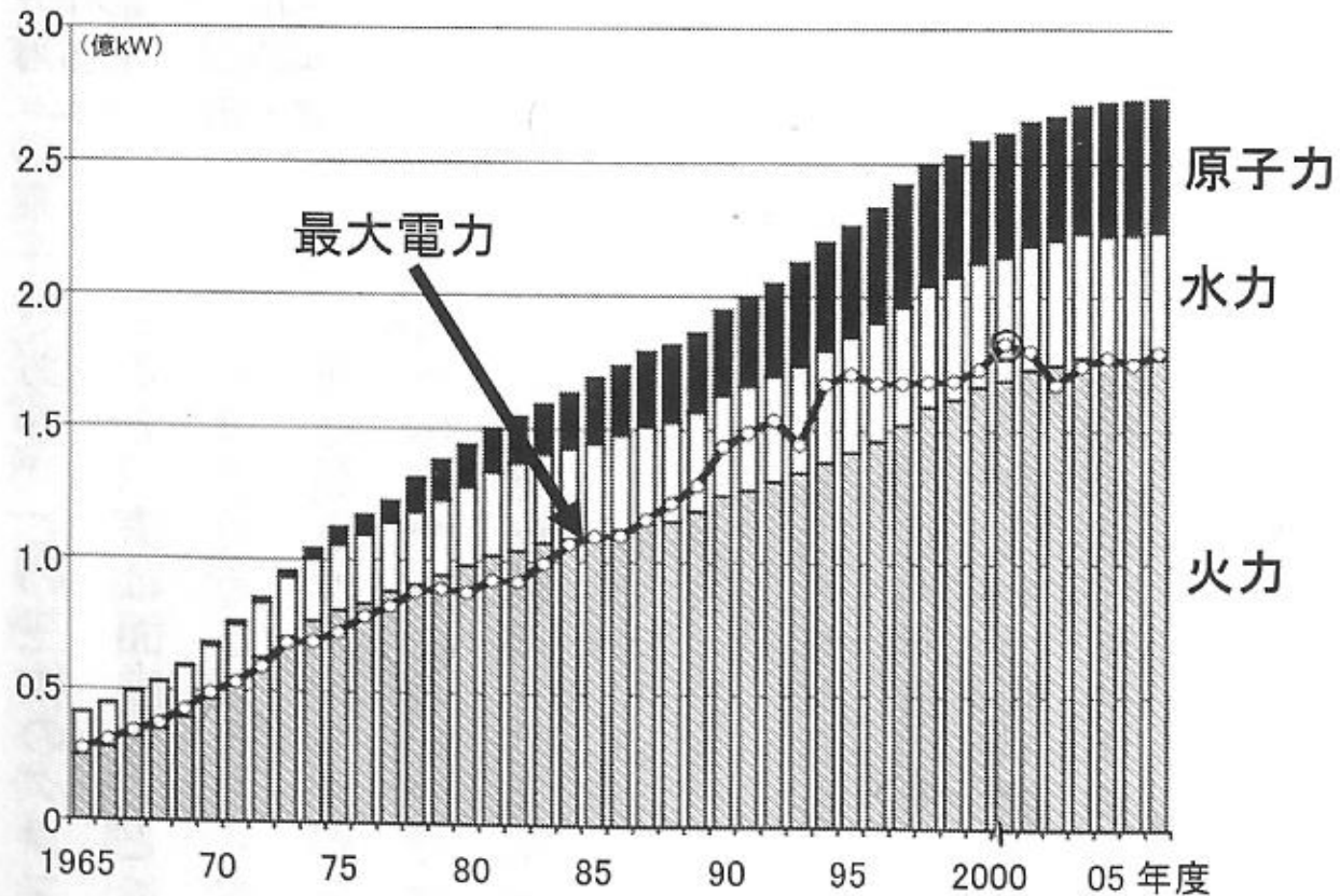
【図64】 発電施設の設備容量と最大電力の推移
